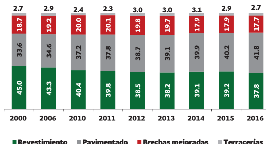
Composición porcentual de la Longitud de la Red Nacional Carretera por estado superficial (Porcentaje)
