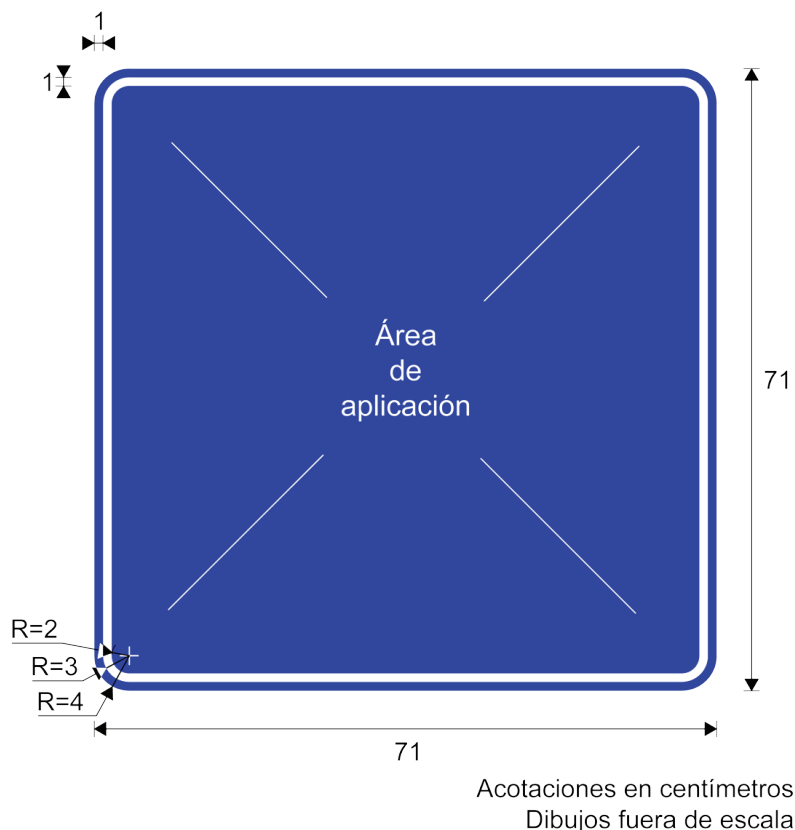
Figura II.5-9. Área de aplicación y dimensiones de los elementos del tablero de las señales turísticas y de servicios
