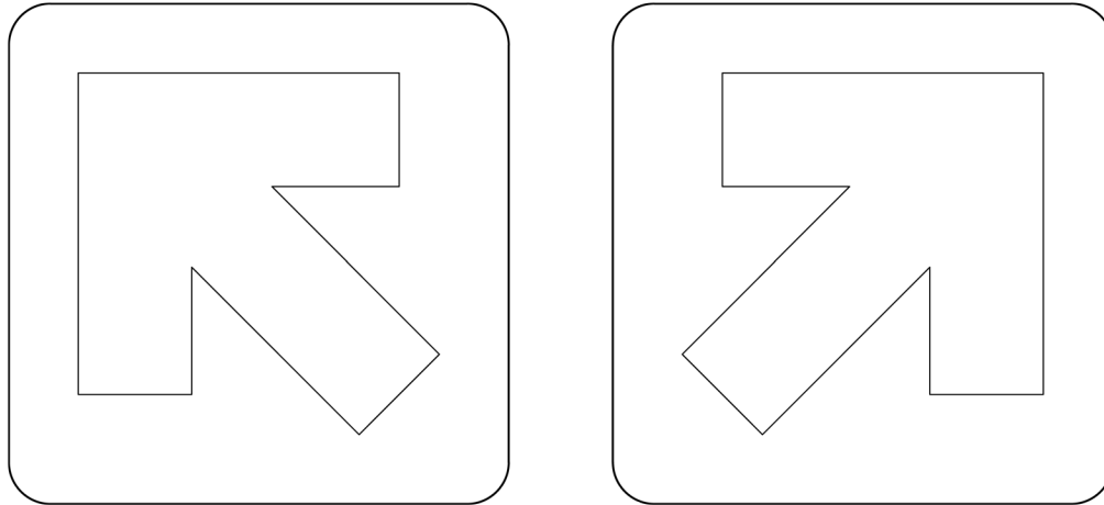
Figura II.5-3. Trazo de flechas diagonales en tableros de flechas complementarias
