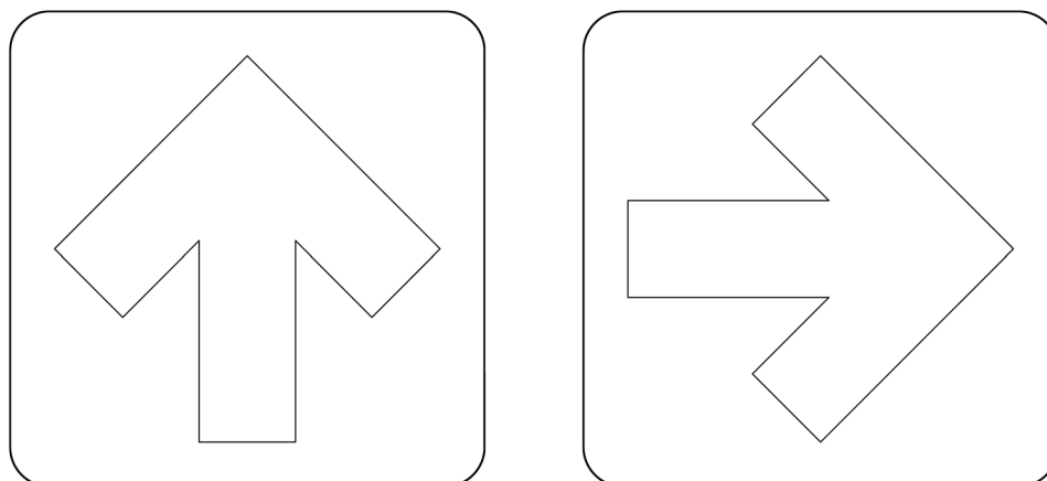
Figura II.5-2. Trazo de flechas horizontal y vertical en tableros de flechas complementarias
