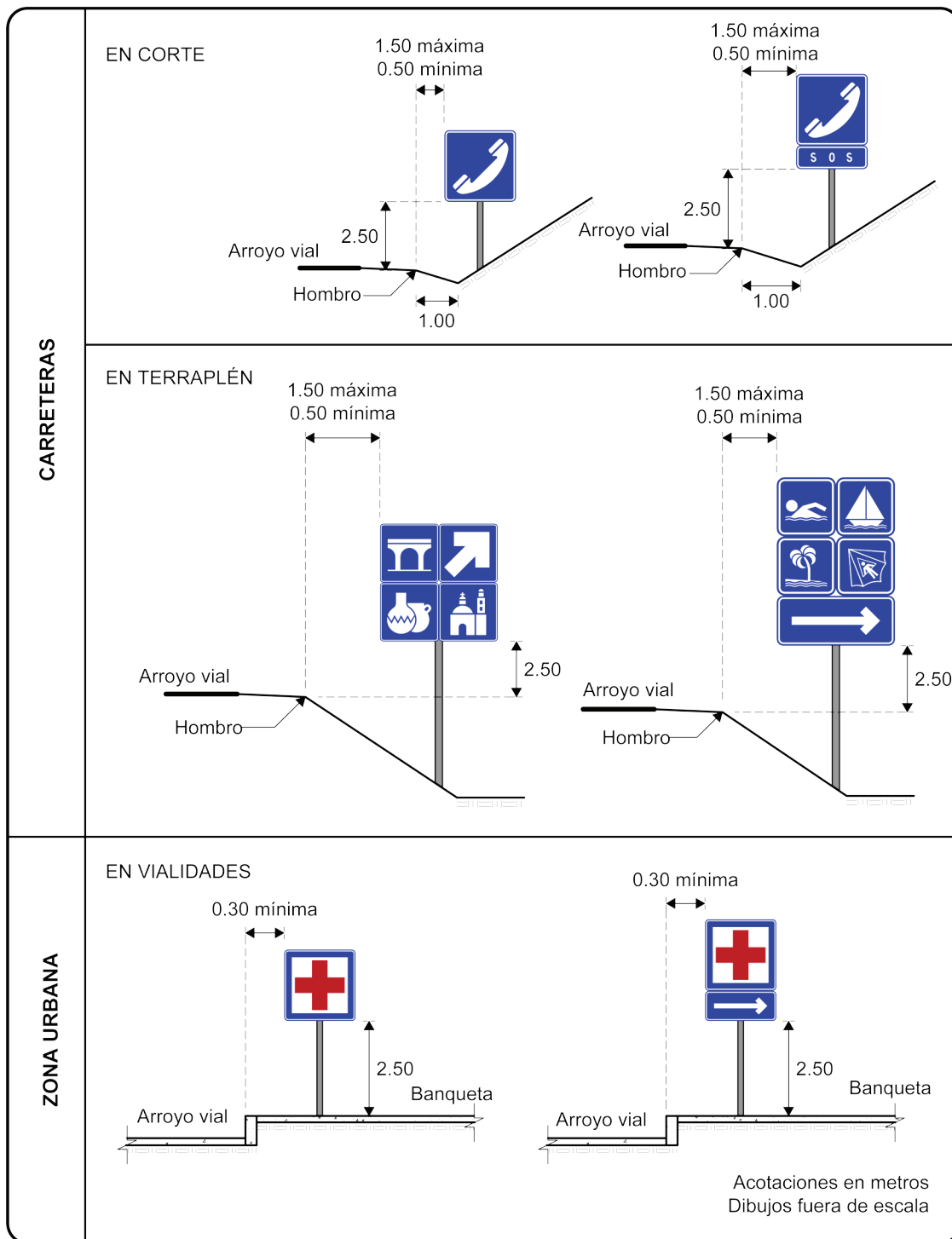
Figura II.5-11. Ejemplo de colocación lateral de las señales turísticas y de servicios
