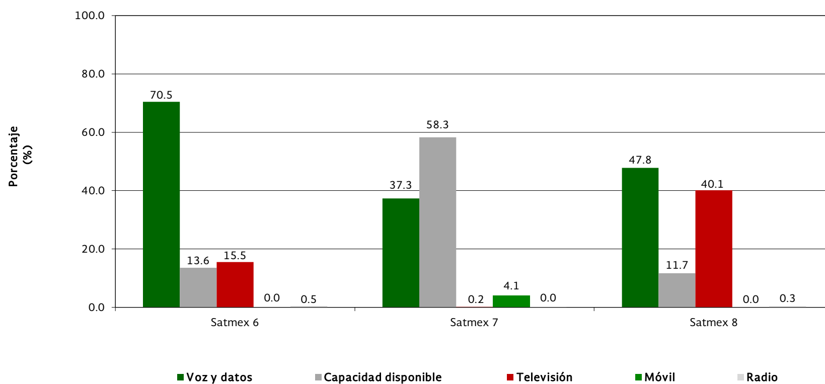
Porcentaje de ocupación del Sistema Mexicano de Satélites por servicio según satélite
