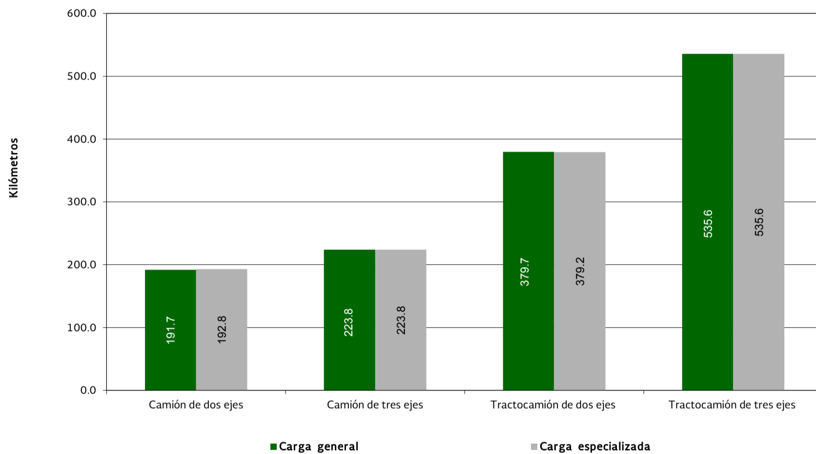
Distancia media recorrida por tonelada transportada según tipo de carga y clase de vehículo
